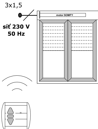
CENTRALIS RTS nástěnný vysílač
